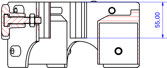
A-A ( 1 : 2 )
